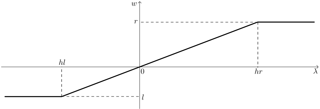
Рис. 1. График функции w(\lambda) .
